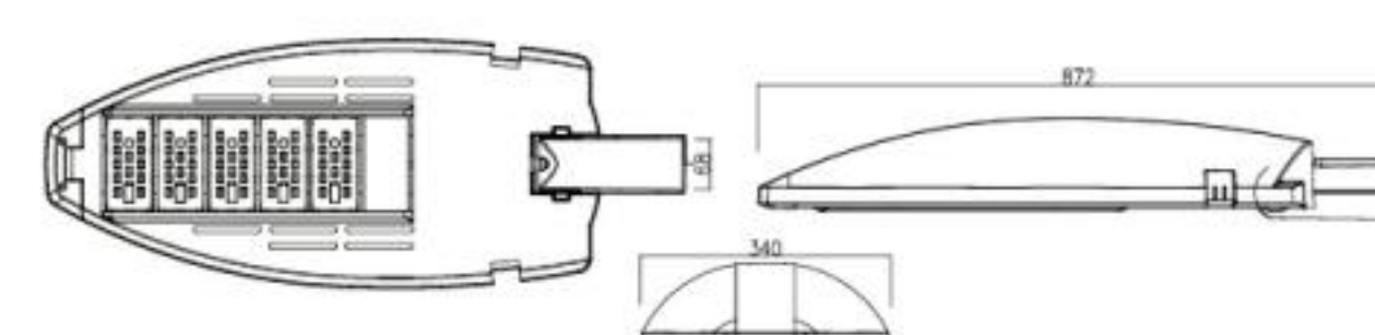
제품도면
