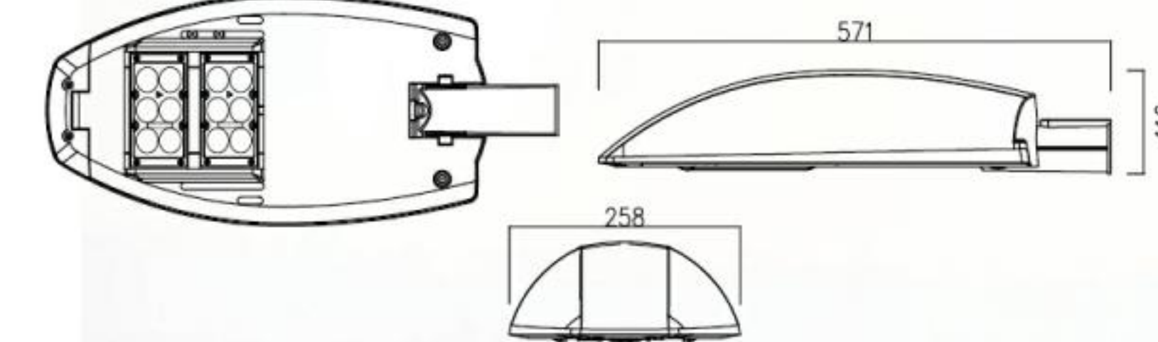
제품도면
