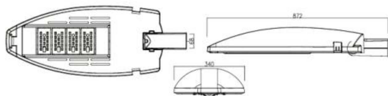
제품도면
