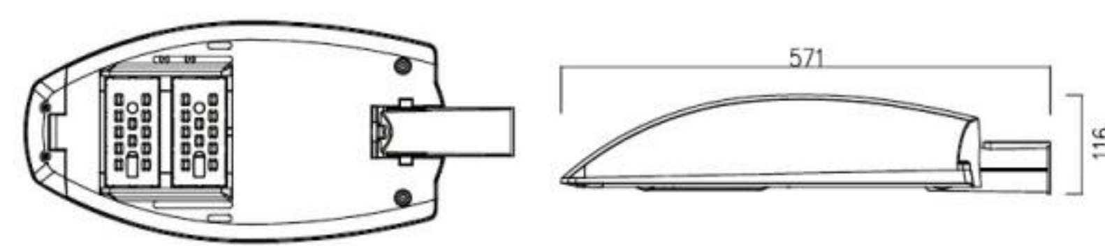
제품도면
