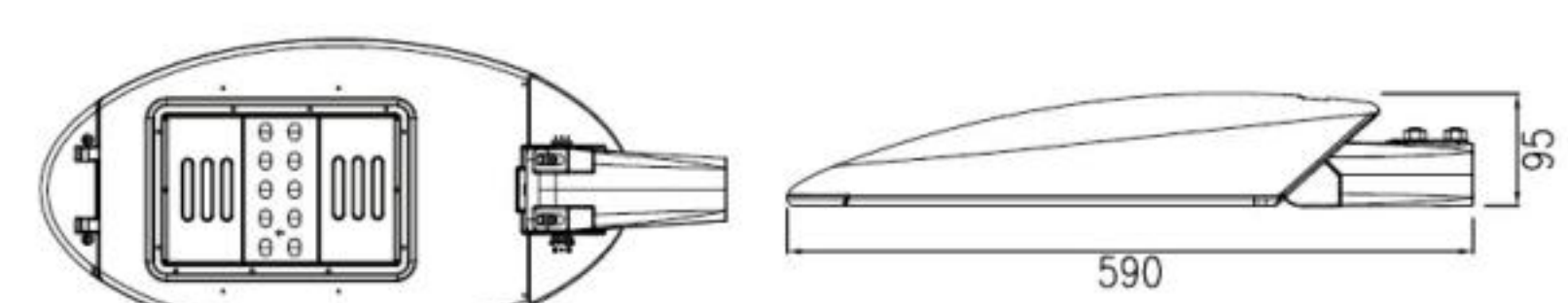
제품도면
