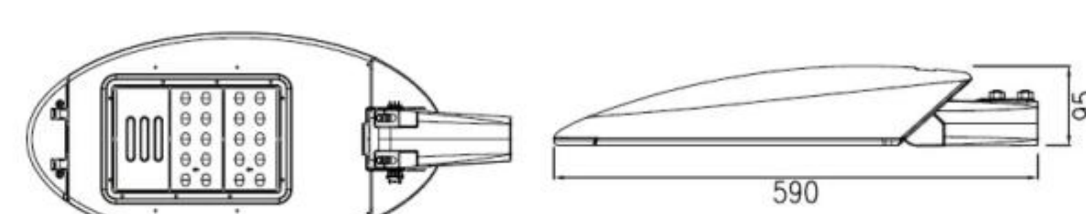
제품도면
