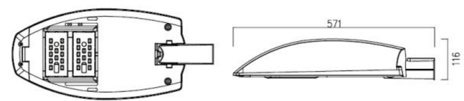
제품도면
